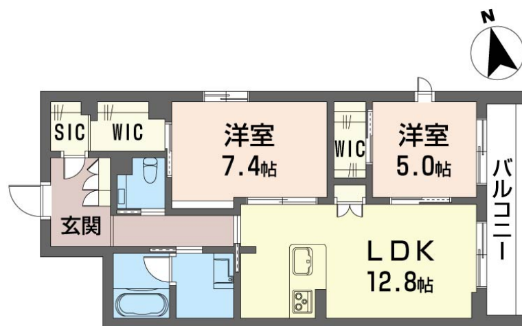
【完成予想図】
